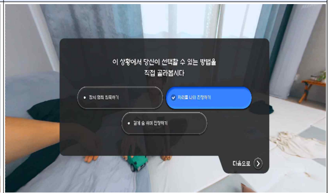
상호 작용(interaction)
